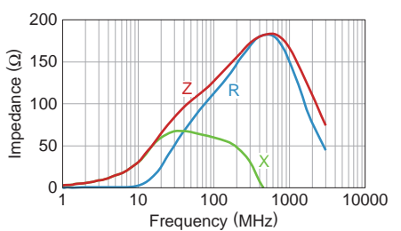
MPZ1608S331ATD25
